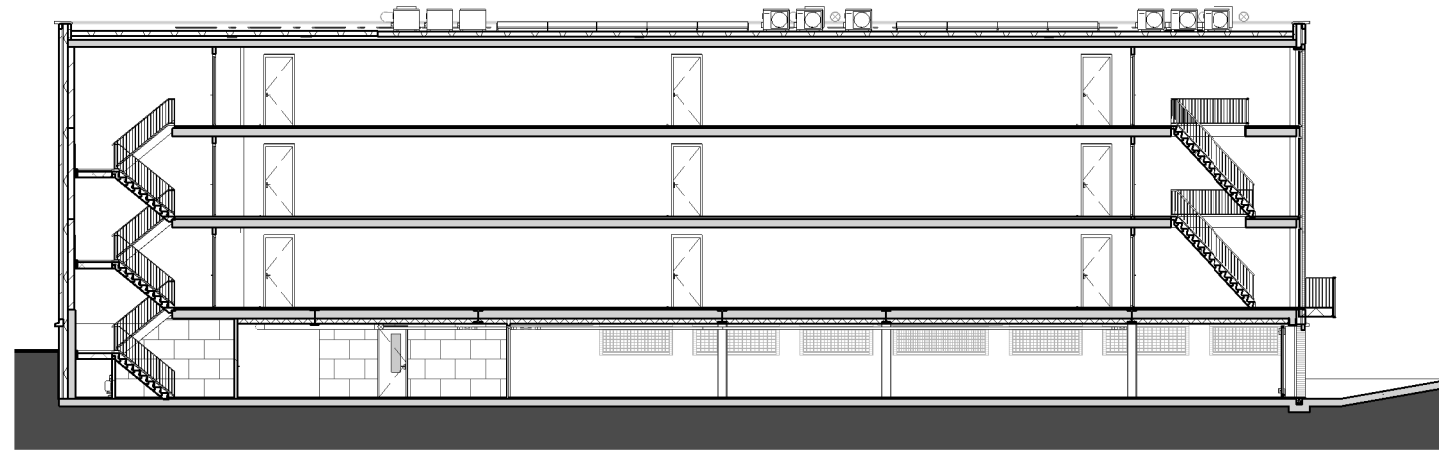
| Langsdoorsnede
